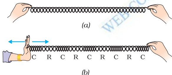
Fig. 12.7: Longitudinal wave in a slinky.
